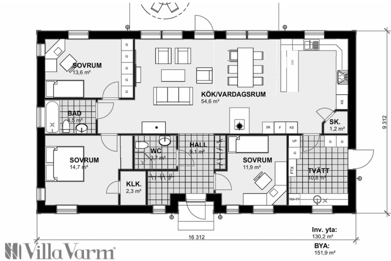
Planlösning Villa Boudden
