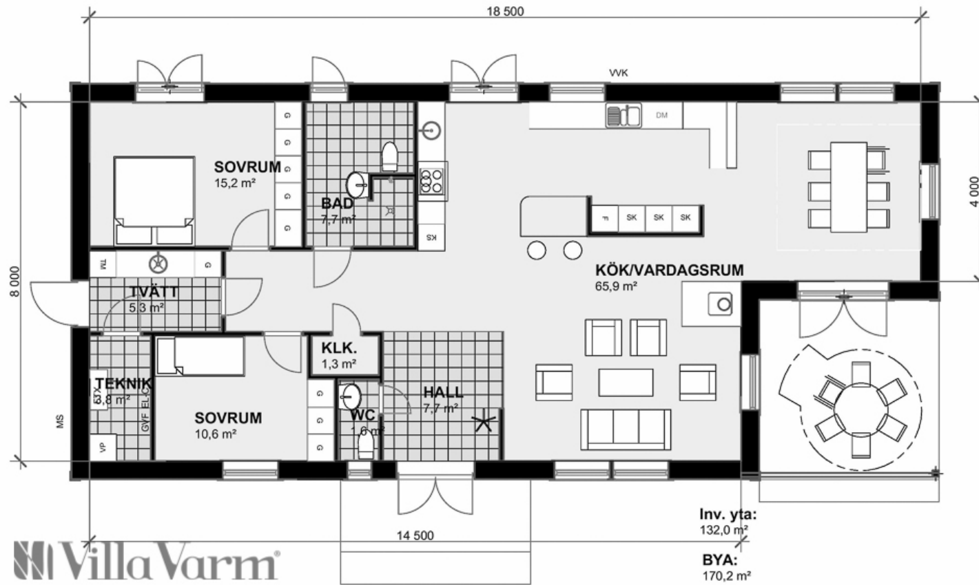
Planlösning Villa Färjestaden
