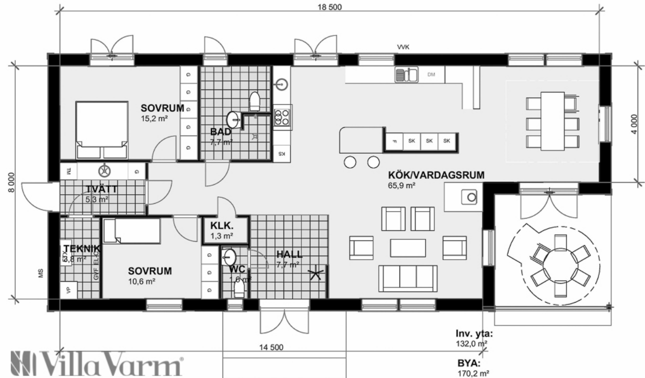
Planlösning Villa Färjestaden
