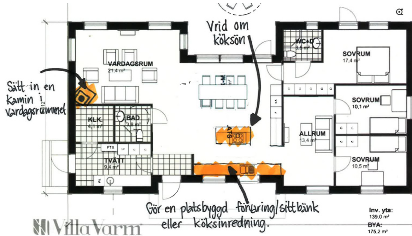
Ändring planlösning Långmyran
