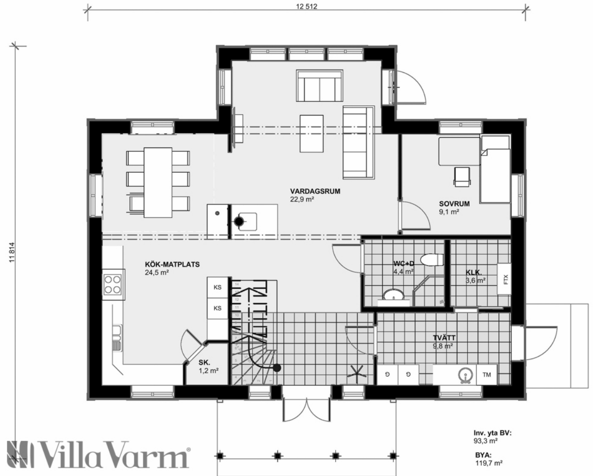
Bottenvåning Villa Nykvarn
